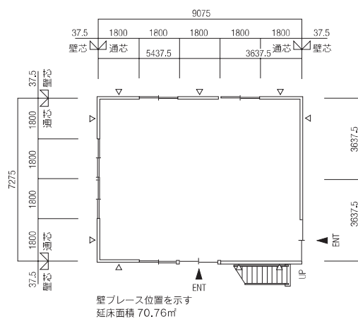
1F 平面図
