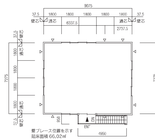
2F 平面図
