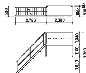
SH-HP型/階段
