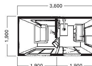
フロハウス B-1型
