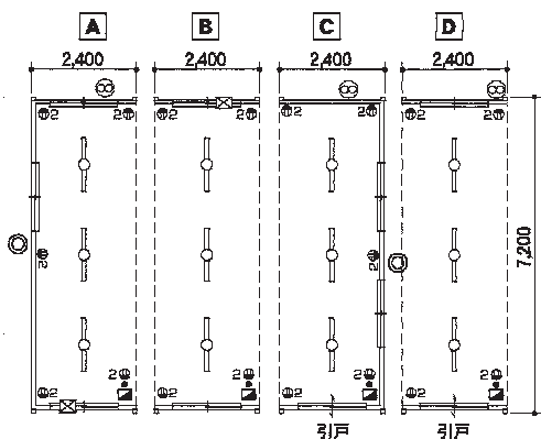
SH-HP72 平面図
