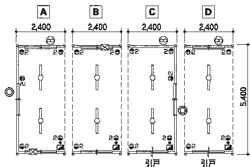
SH-HP54 平面図
